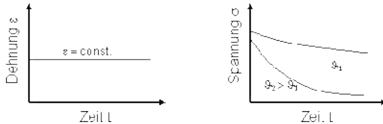
Bild 1: Relaxation von Kunststoffen: Bei konstanter Dehnung fällt die Spannung zeit- und temperatur ( \vartheta )-abhängig ab.
